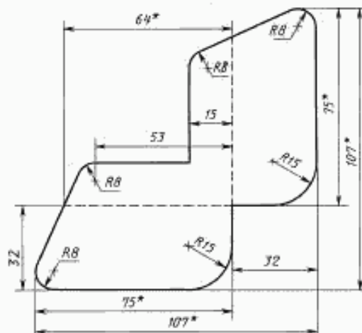
Развертка угольника
